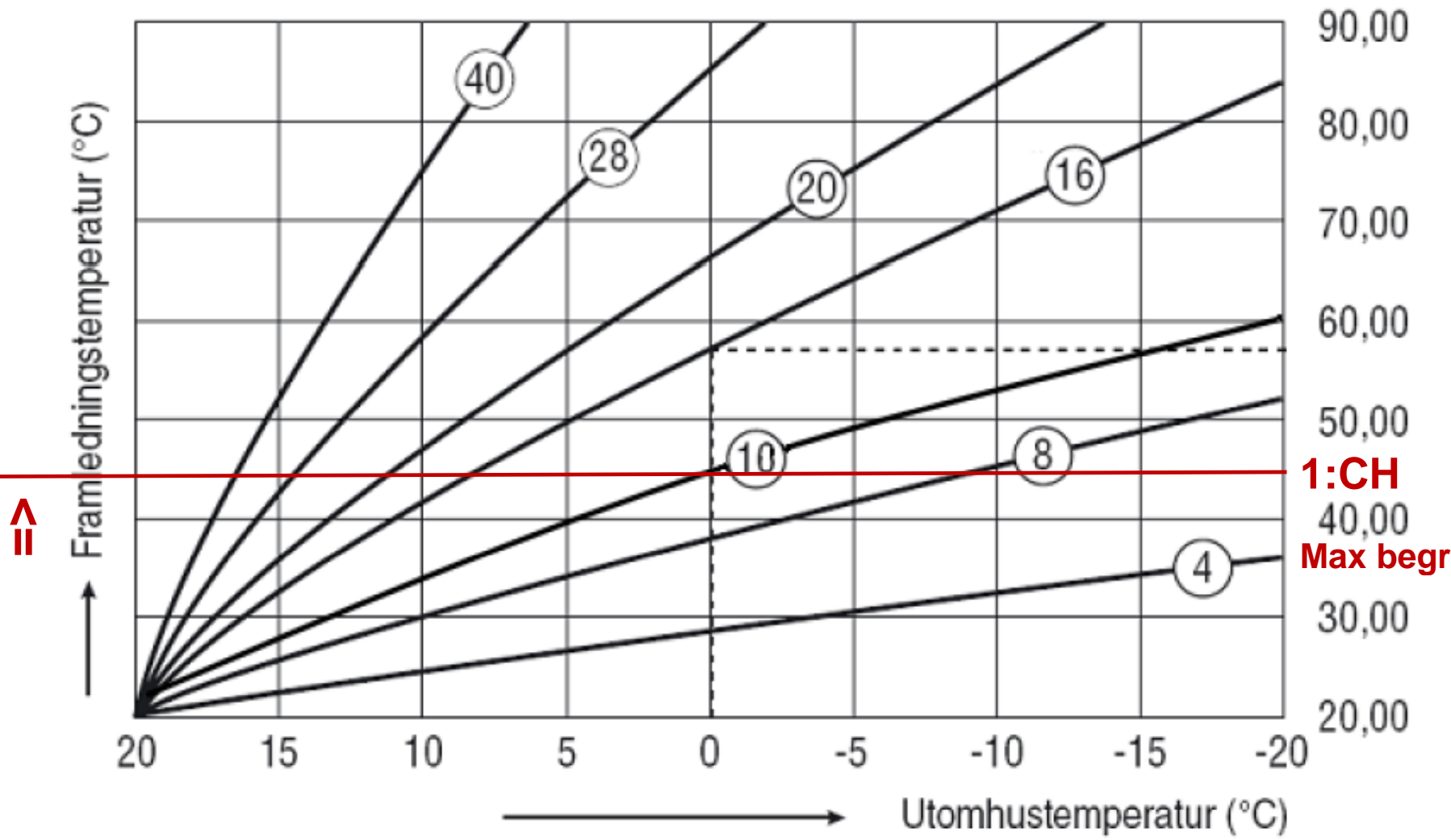
Kurvlutning vid 20°C önskad rumstemperatur.
